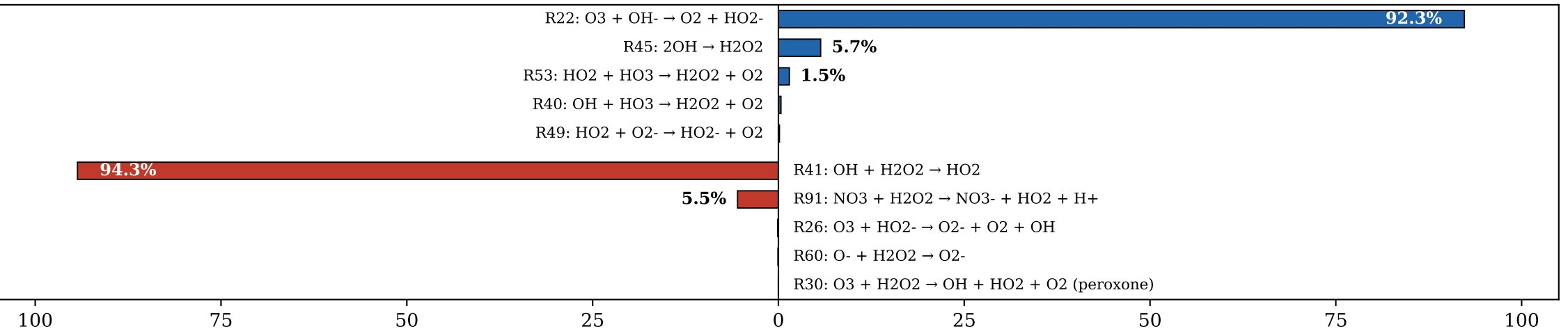
(d) H 2 O 2 (Σsrc = 2.31e-12 M/s)
